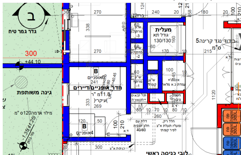
2.2.3 תכנית קומה טיפוסית: לובי כניסה ראשי
